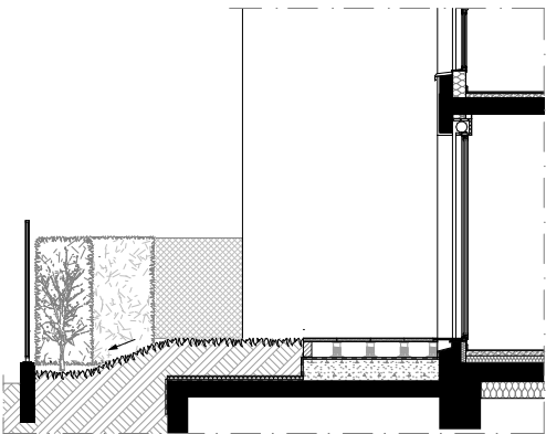
COUPE DE PRINCIPE SUR TERRASSE ET JARDIN
