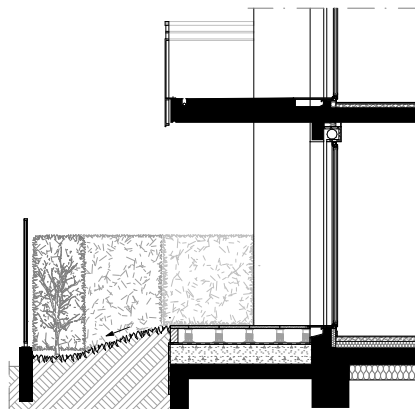
COUPE DE PRINCIPE SUR TERRASSE ET JARDIN
