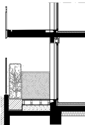
COUPE DE PRINCIPE SUR TERRASSE ET JARDIN
