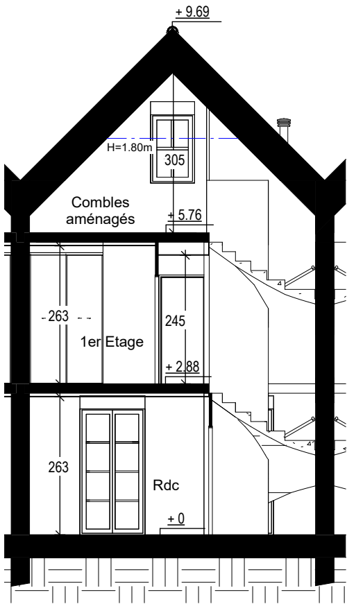
COUPE
