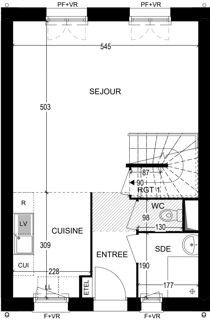
REZ-DE-CHAUSSEE
