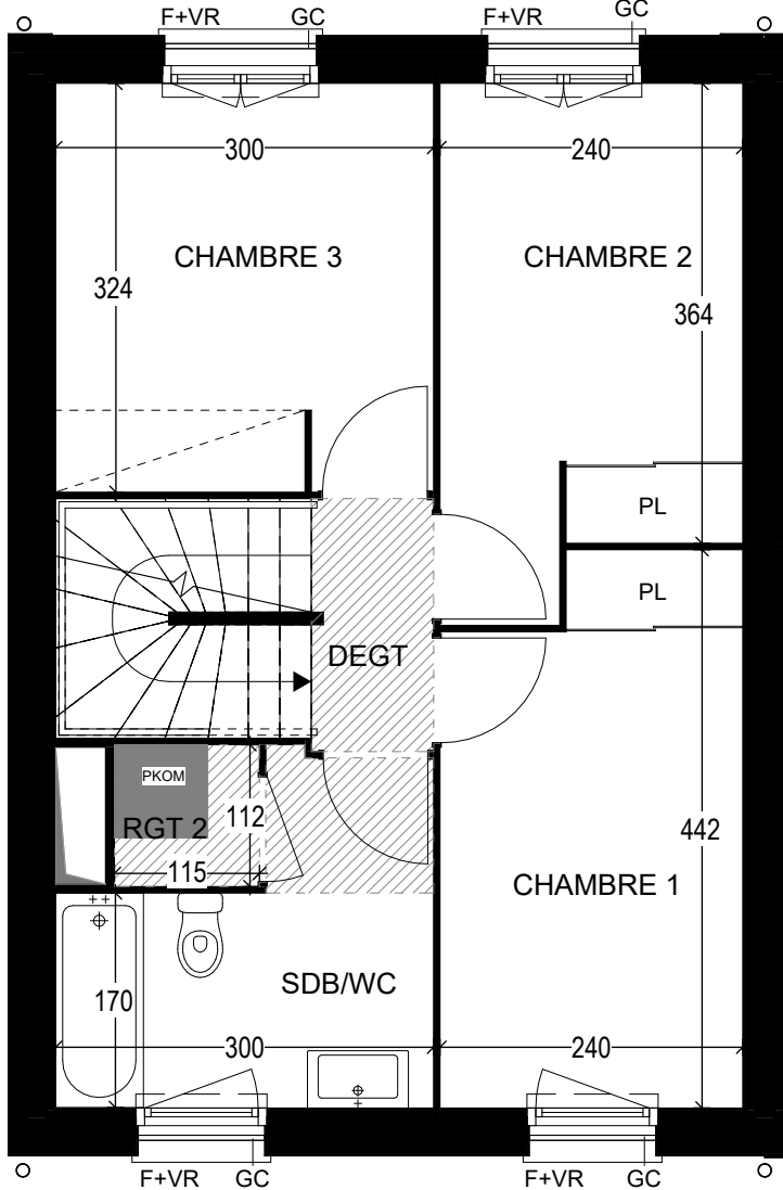
ETAGE
