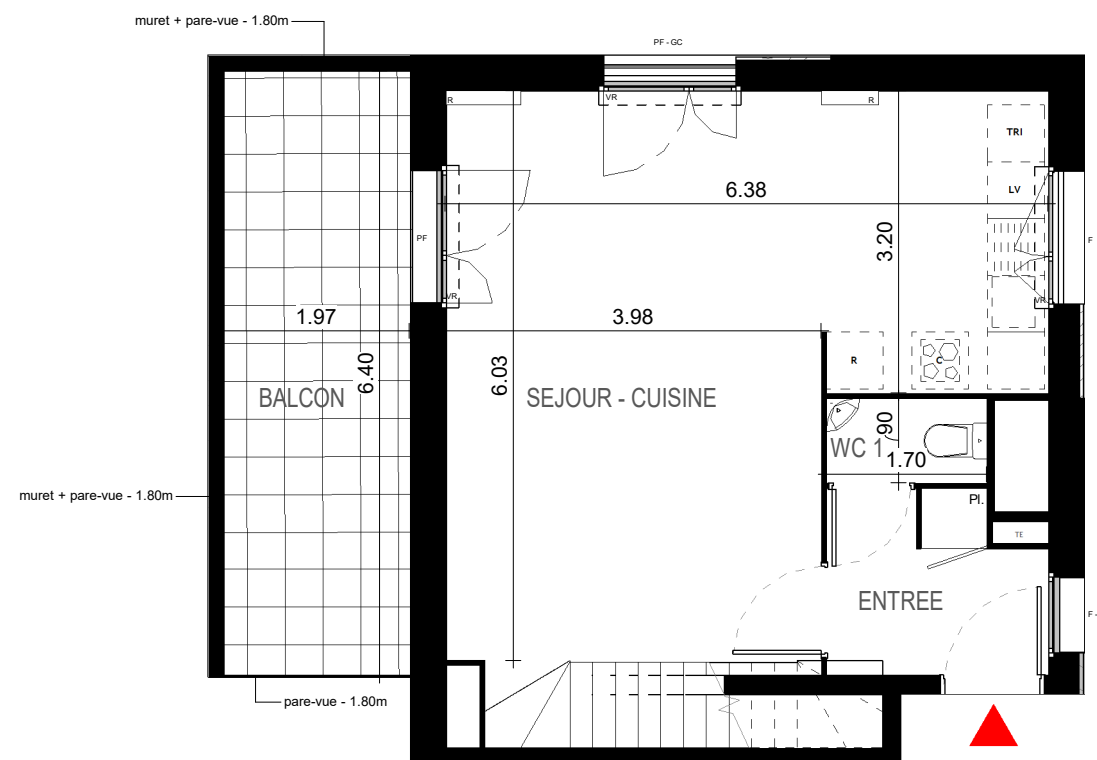
1ER ETAGE
