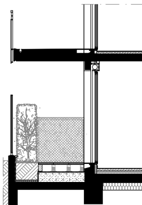
COUPE DE PRINCIPE SUR TERRASSE ET JARDIN
