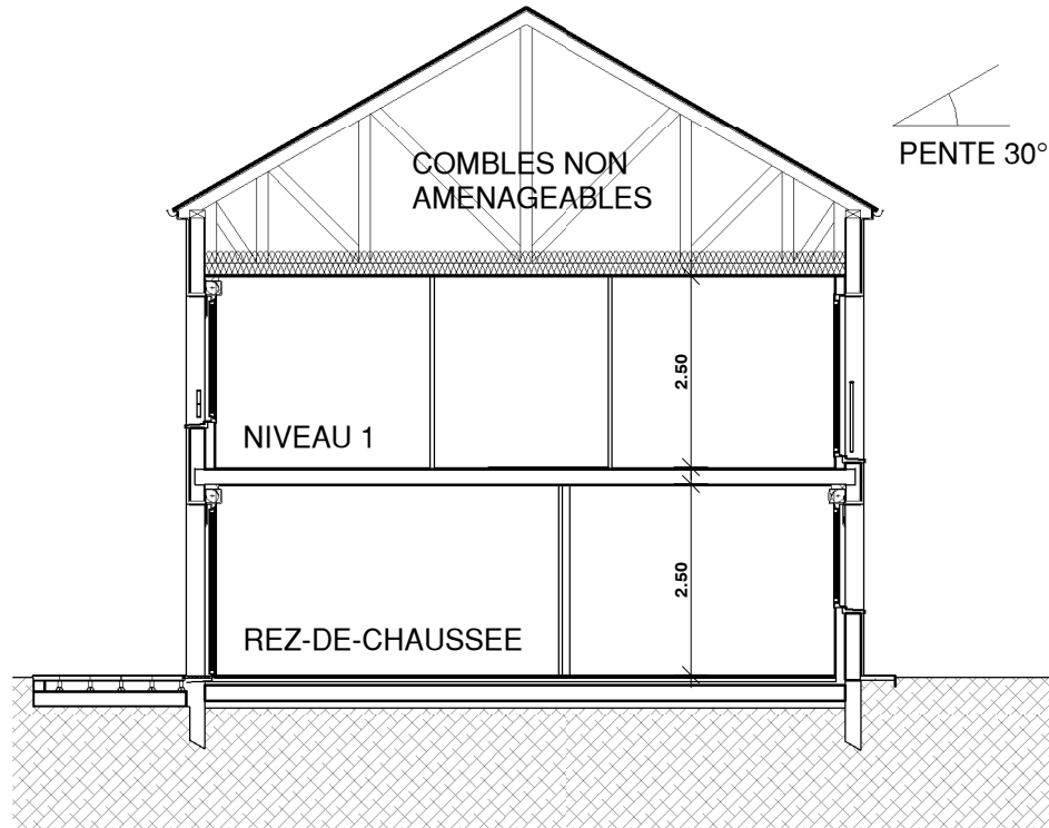
COUPE
