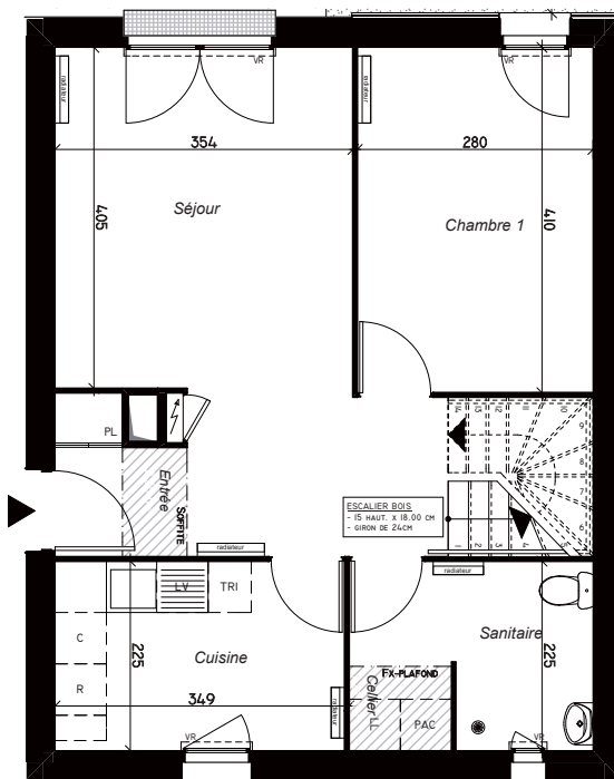
REZ-DE-CHAUSSEE
