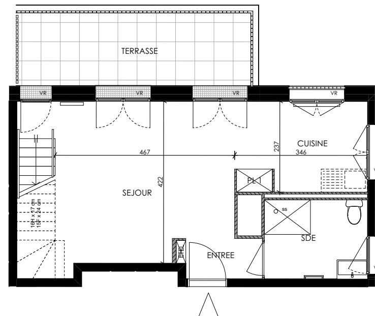
NIVEAU BAS
