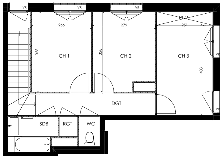
NIVEAU HAUT
